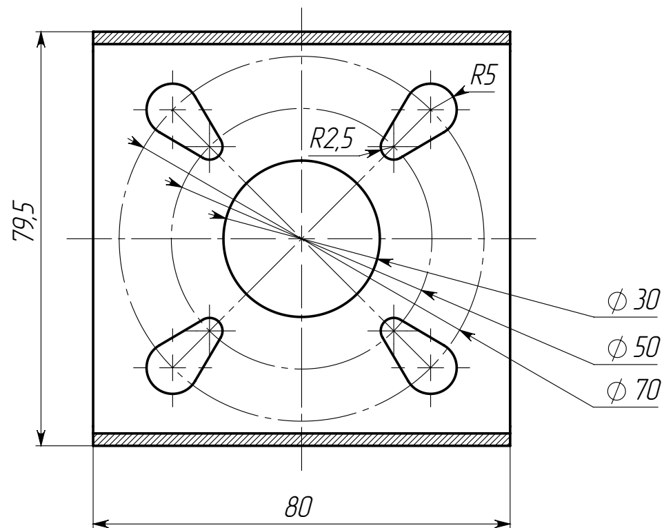
A-A (1 : 1)
